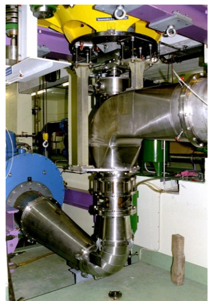
Photo de la turbine axiale montée sur le stand d'essai Mhylab
